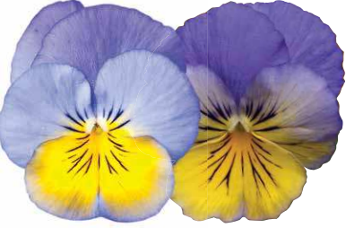
Morpho
